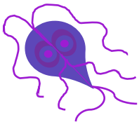
Schema-Zeichnung Trophozoit
